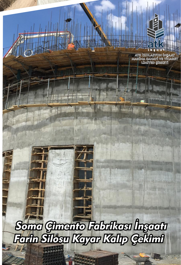
Soma Çimento Fabrikası İnşaatı Farin Silosu Kayar Kalıp Çekimi
